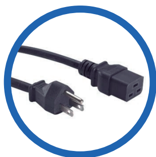
Conectores NEMA 5-15P / IEC-C19
