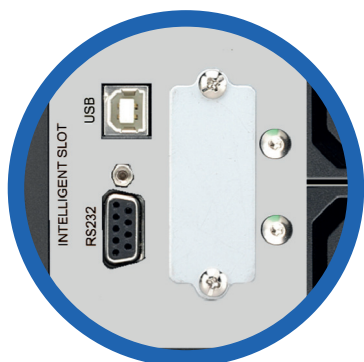
Conector para banco de baterías externo y puertos de comunicación USB y R232
