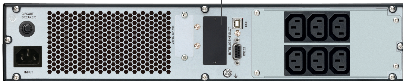
6 terminales IEC-13
