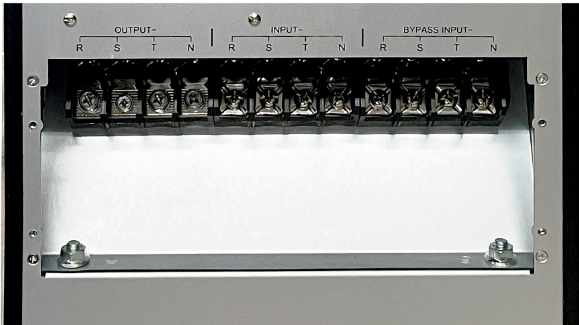
Block de terminales entrada/salida
