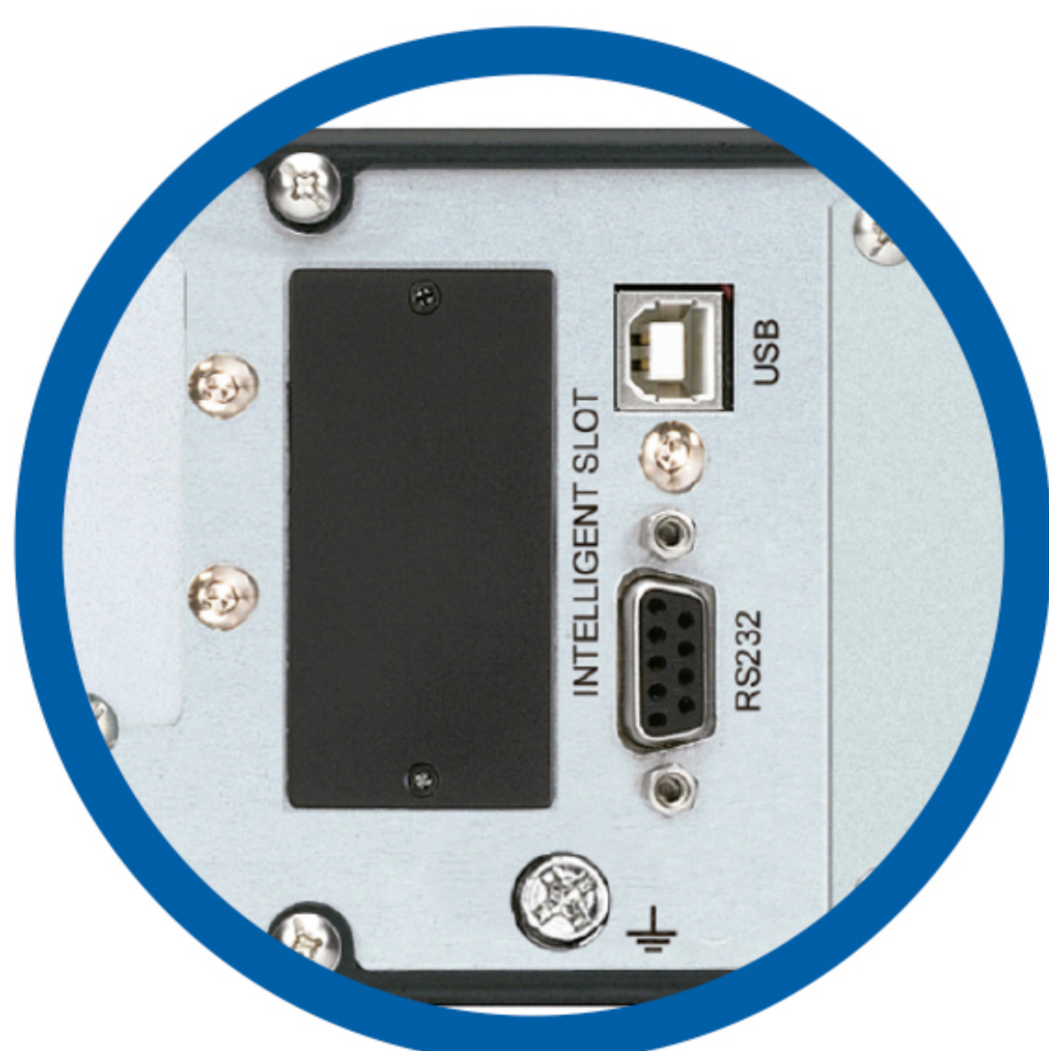
Slot para tarjetas inteligentes y puertos de comunicación USB y R232
