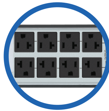
8 terminales de salidas NEMA 5-15R o 5-20R
