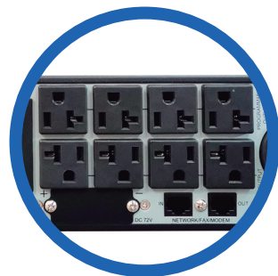
8 terminales de salida NEMA 5-15R o NEMA 5-20R, de los cuales 4 son programables
