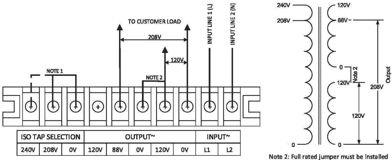
Figura Cableado de salida: 208 V y 120 V
