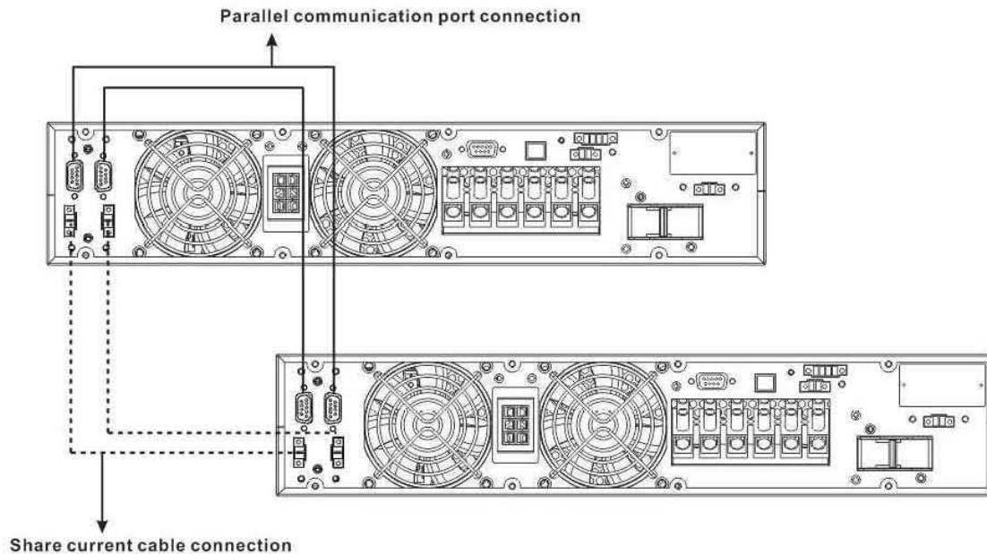
Diagrama 4: Diagrama de cableado del sistema paralelo
