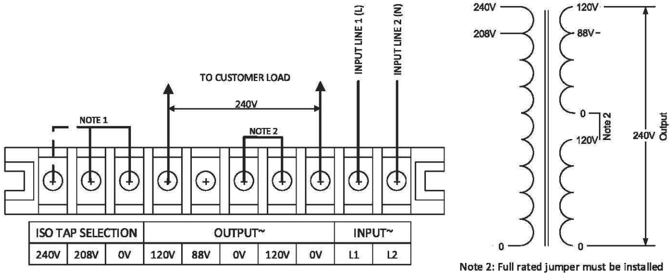
Figura Cableado de salida: 240 V
