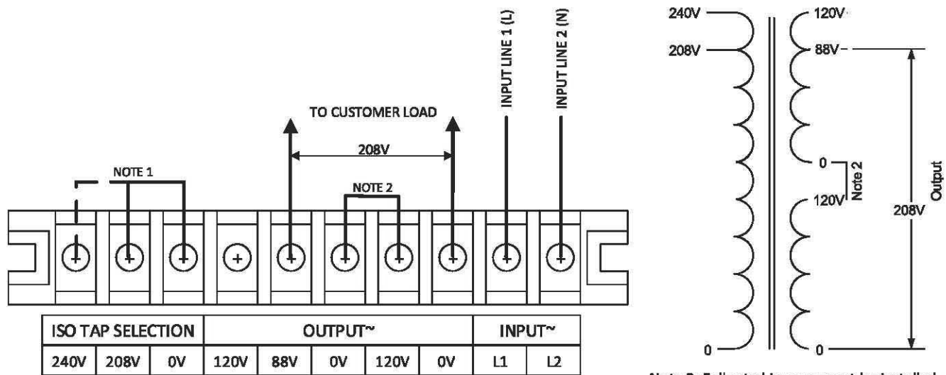
Figura Cableado de salida: 208 V
