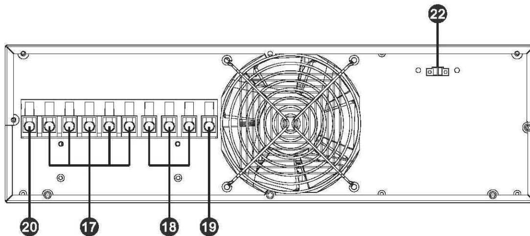
Diagrama 5: Terminal de salida del paquete ISO
